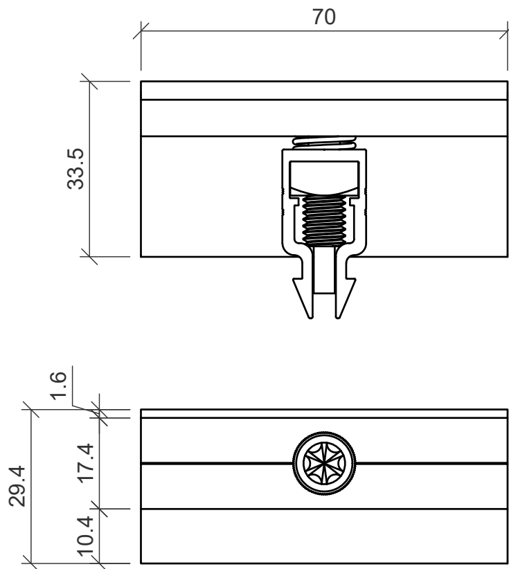
M8 Zylinderschraube
