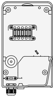
Anschlussdose
